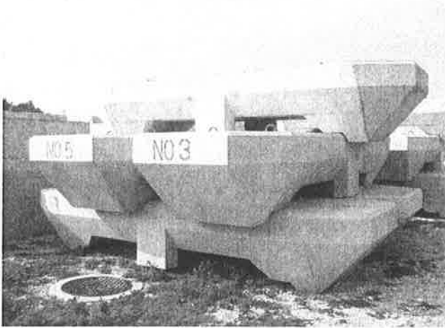
多目的藻礁の製作及び設置状況
