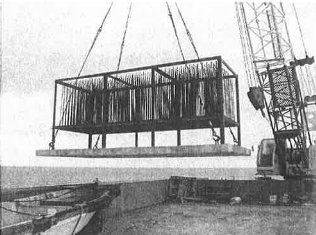
アオリイカ産卵礁の設置状況
